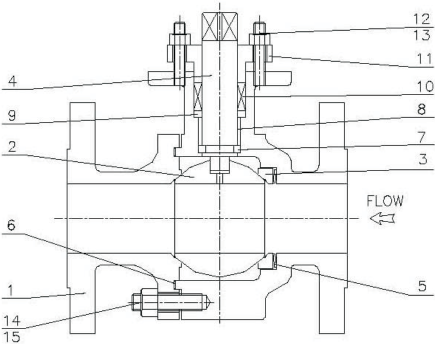
图1-1 阀本体结构 Fig 1-1 Valve Structure 浮动球形式 Floating Type Dn100及以下尺寸 4" And Under 有流向要求 With Flow Dir. Req.
