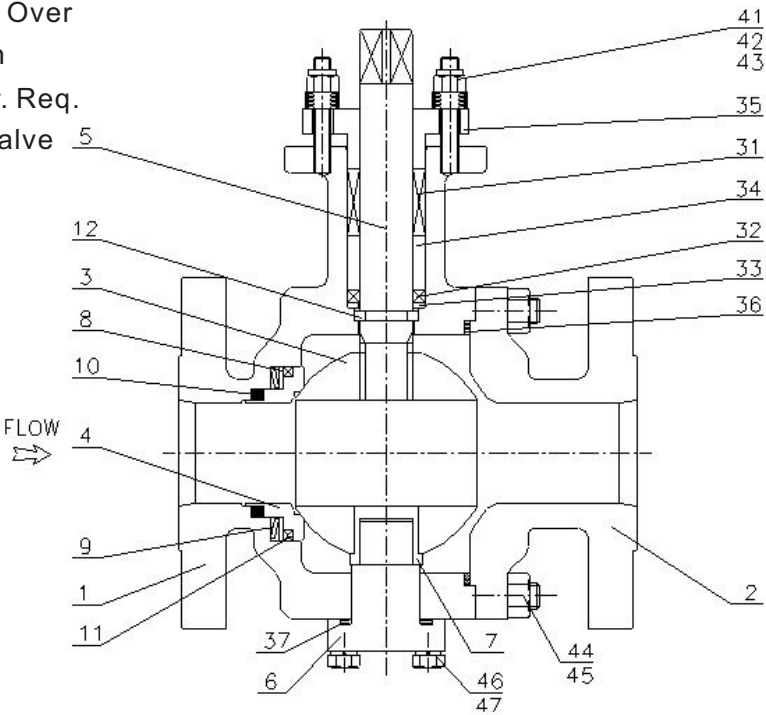
图1-4 阀本体结构 Fig 1-4 Valve Structure
